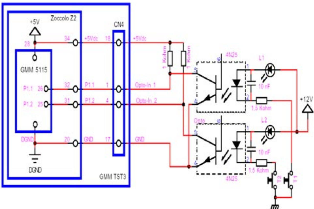
Schema Applicativo per Ingressi Optoisolati del Tipo NPN.
