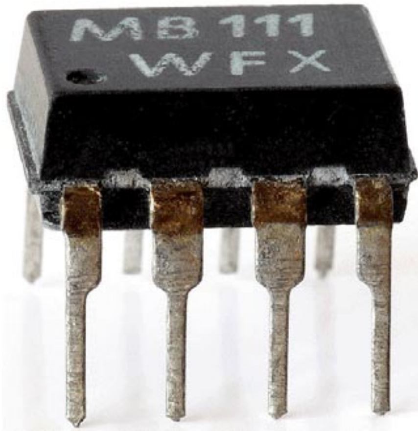
Un tipico Optoisolatore in un Contenitore DIL a 4+4 piedini.
