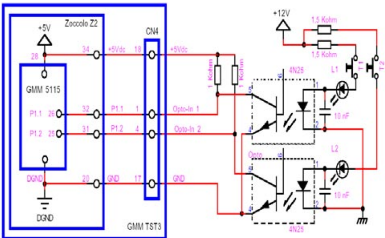
Schema Applicativo per Ingressi Optoisolati del Tipo PNP.
