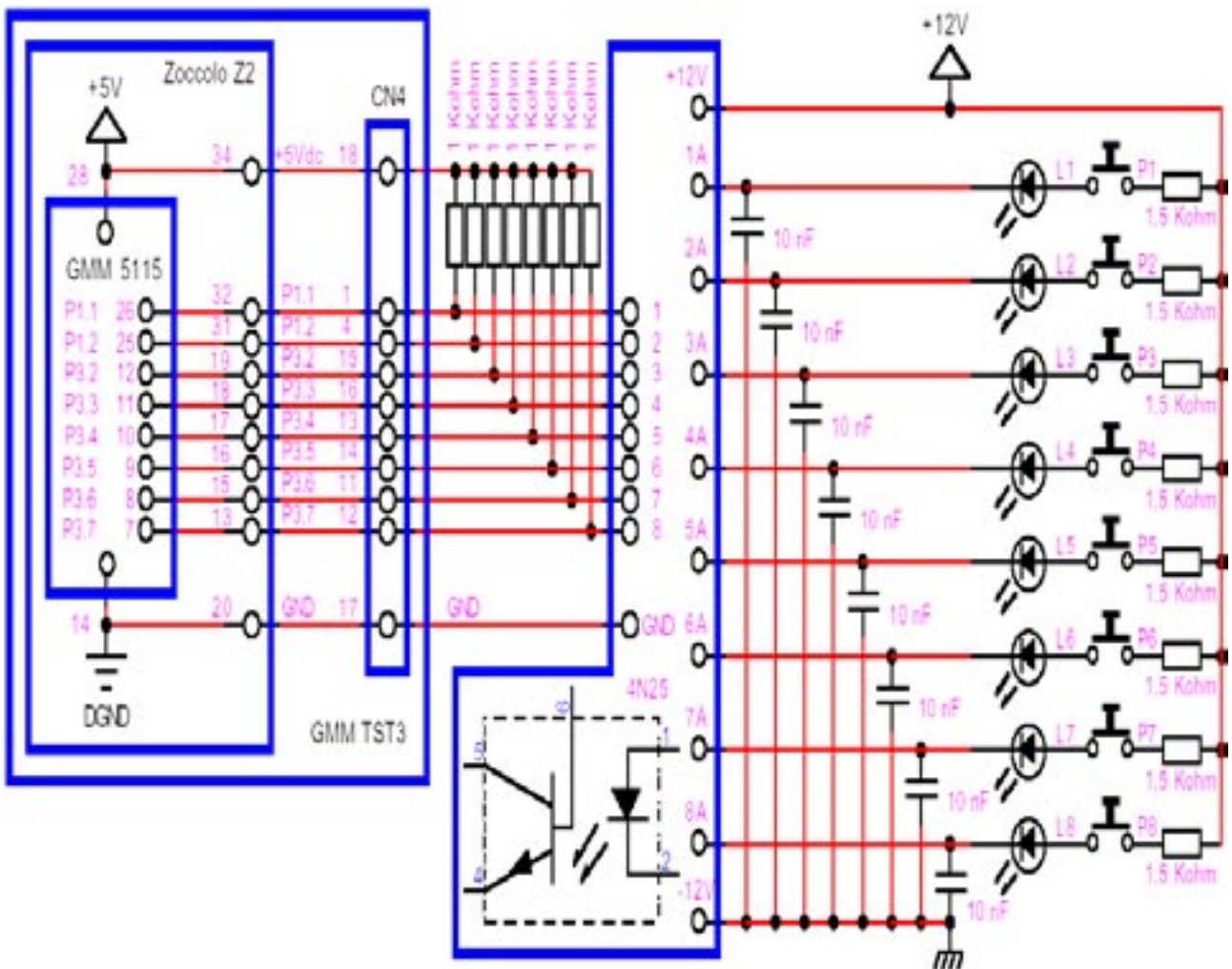
Schema Applicativo per 8 Ingressi Optoisolati del Tipo PNP.
