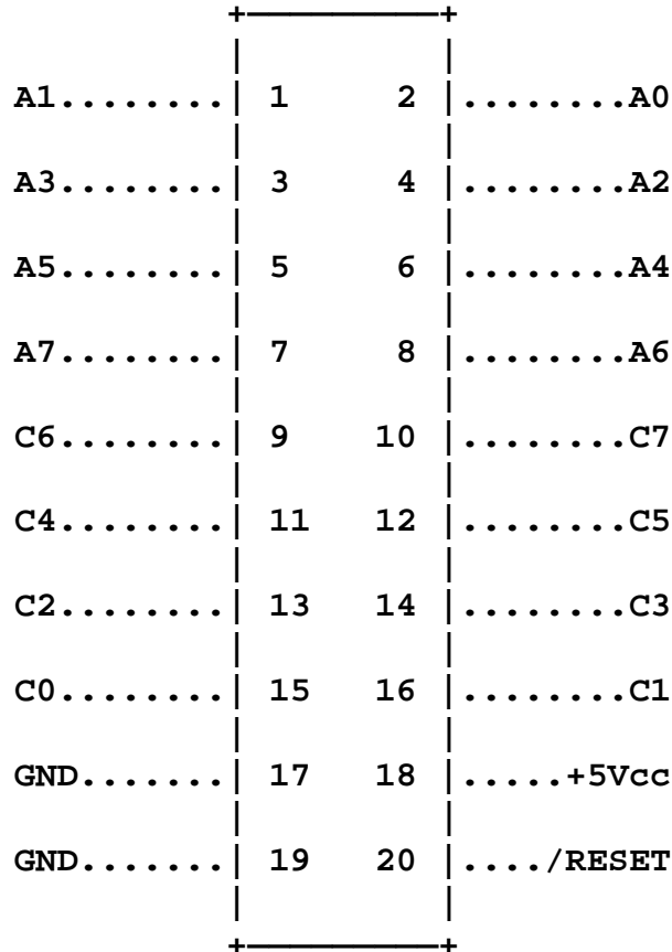
Fig. 4-5: Connettore CN5.
