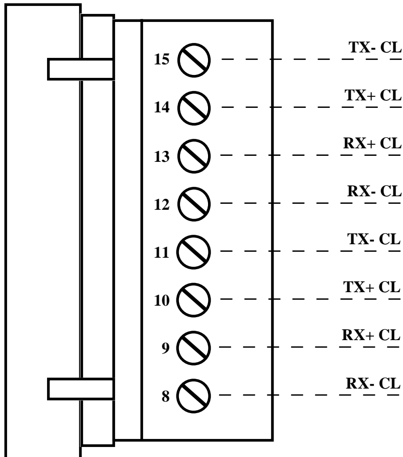
FIGURA 6: CN5 CONNETTORE 2 LINEE SERIALI IN C. L. ATTIVE SU NNI 16
